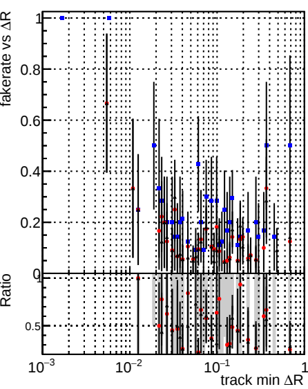
Legend: DOMstep3_TT_CKF (blue dots), DOMstep3_TT_default (red dots), DOMstep3_TT_defaultNEW2 (black dots)
