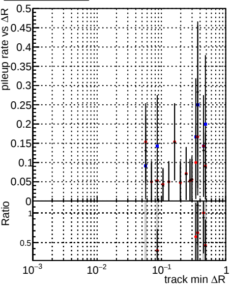
Legend: DOMstep3_TT_CKF (blue dots), DOMstep3_TT_default (red dots), DOMstep3_TT_defaultNEW2 (black dots)
