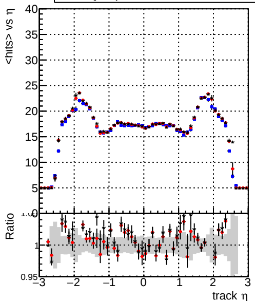
mean hits vs \eta — DQMstep3_TT_CKF — DQMstep3_TT_default — DQMstep3_TT_defaultNEWT2
