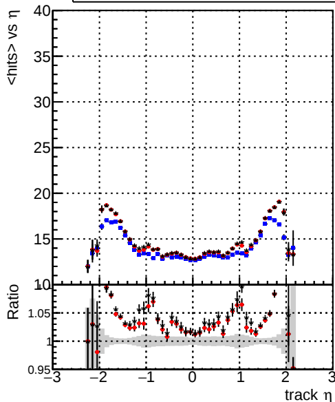
mean hits vs \eta — DQMstep3_TT_CKF — DQMstep3_TT_default — DQMstep3_TT_defaultNEWT2
