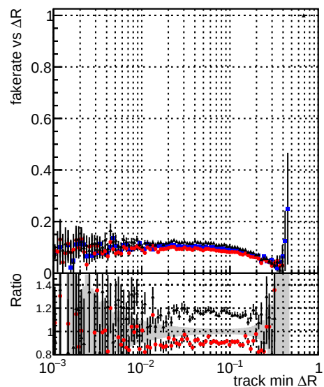
—●— DQMstep3_TT_CKF —●— DQMstep3_TT_default —●— DQMstep3_TT_defaultNEW2
