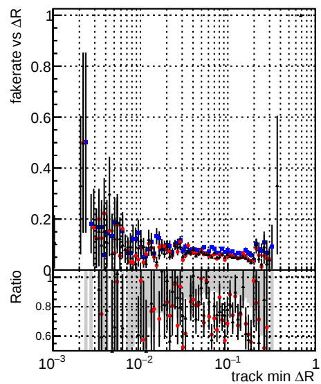
Legend: DQMstep3_TT_CKF (blue diamonds) DQMstep3_TT_default (red circles) DQMstep3_TT_defaultNEW2 (black crosses)
