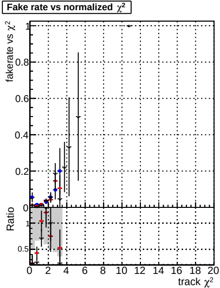
Fake rate vs. DOMstep3 CKF DOMstep3 default DOMstep3 defaultNEWT3
