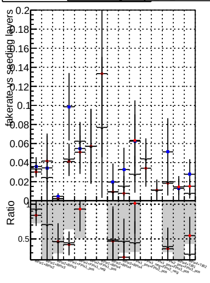
Fake rate vs. DOMstep3 CKF DOMstep3 default DOMstep3 defaultNEWT3
