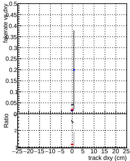
Fake rate vs d DOMstep3 TT CKF DOMstep3 default DOMstep3 defaultNEWT3
