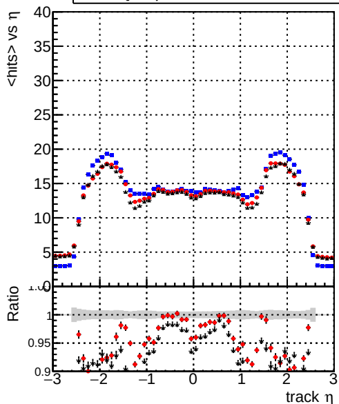
DQMstep3_TT_CKF DQMstep3_TT_default DQMstep3_TT_defaultNEWT3 mean hits
