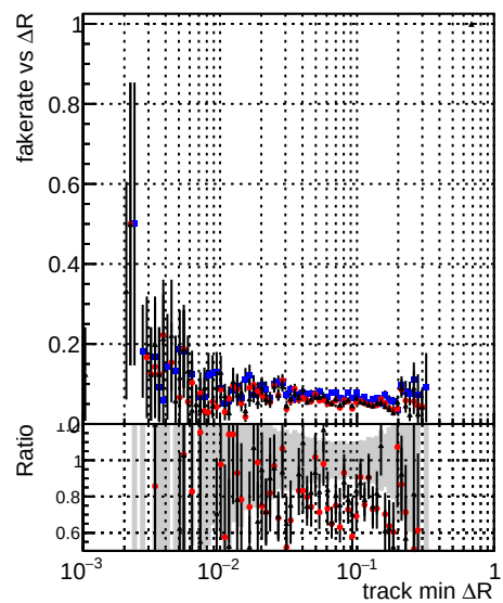
—●— DQMstep3 TT CKF —●— DQMstep3 TT default —●— DQMstep3 TT defaultNEW3
