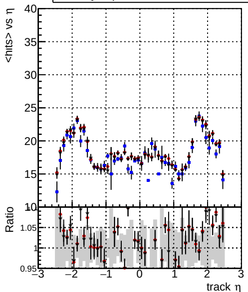
mean hit — DQMstep3_TT_CKF — DQMstep3_TT_default — DQMstep3_TT_defaultNEWT3
