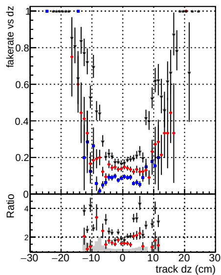
Fake rate vs d DOMstep3 CKF DOMstep3 default default NEWT3
