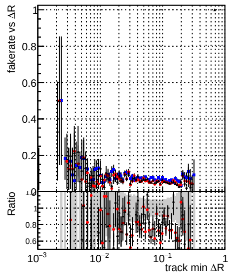
Legend: DQMstep3 TT CKF (blue circles) DQMstep3 TT default (red circles) DQMstep3 TT defaultNEW3 (black circles)
