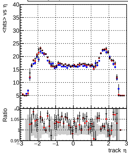
mean hits vs \eta — DQMstep3_TT_CKF — DQMstep3_TT_default — DQMstep3_TT_defaultNEWT3
