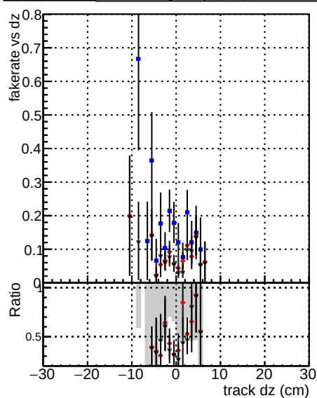
—•— DOMstep3 TT CKF —•— DOMstep3 TT default —•— DOMstep3 TT defaultNEWT3
