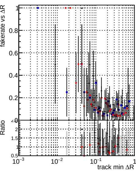
Legend: DQMstep3 TT CKF (blue), DQMstep3 TT default (red), DQMstep3 TT defaultNEW3 (black)
