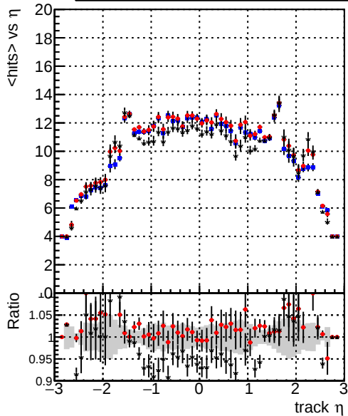
mean hit — DQMstep3_TT_CKF — DQMstep3_TT_default — DQMstep3_TT_defaultNEWT3
