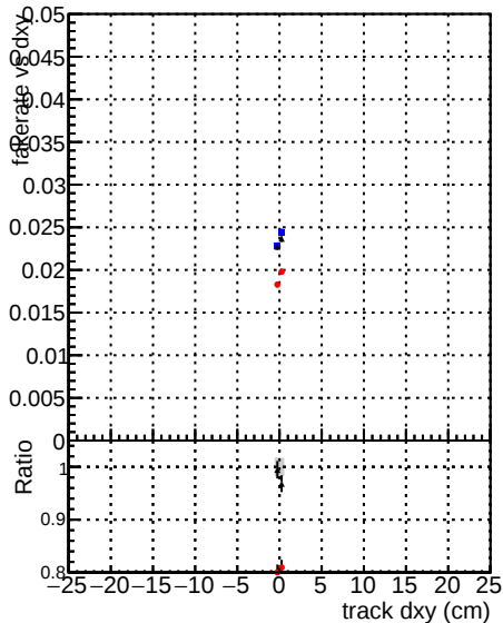
—•— DOMstep3 TT CKF —•— DOMstep3 TT default —•— DOMstep3 TT NEWT3
