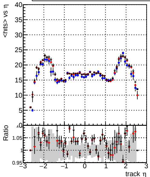
mean hits — DQMstep3_TT_CKF — DQMstep3_TT_default — DQMstep3_TT_defaultNEWT3
