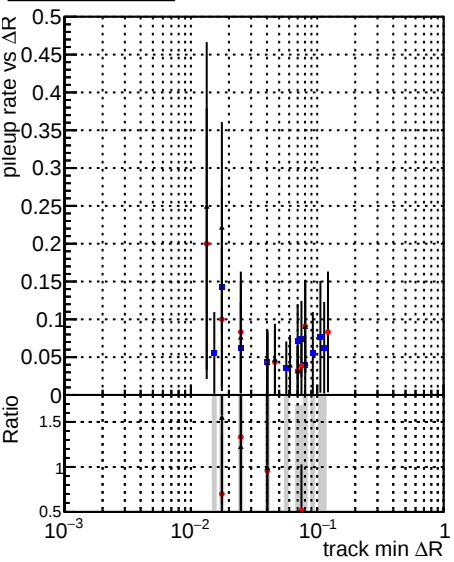
Legend: DQMstep3_TT_CKF (blue dots), DQMstep3_TT_default (red dots), DQMstep3_TT_defaultNEW3 (black line)
