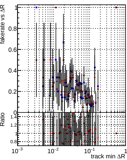
Legend: DQMstep3_TT_CKF (blue dots), DQMstep3_TT_default (red dots), DQMstep3_TT_defaultNEW3 (black line)
