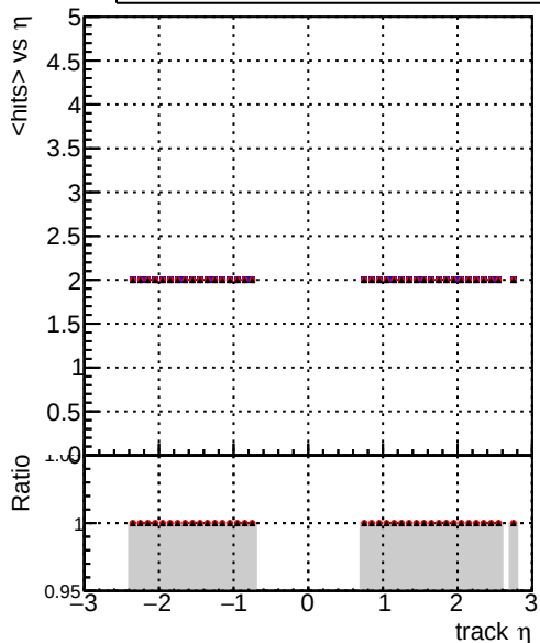
mean hit — DQMstep3_TT_CKF — DQMstep3_TT_default — DQMstep3_TT_defaultNEWT203
