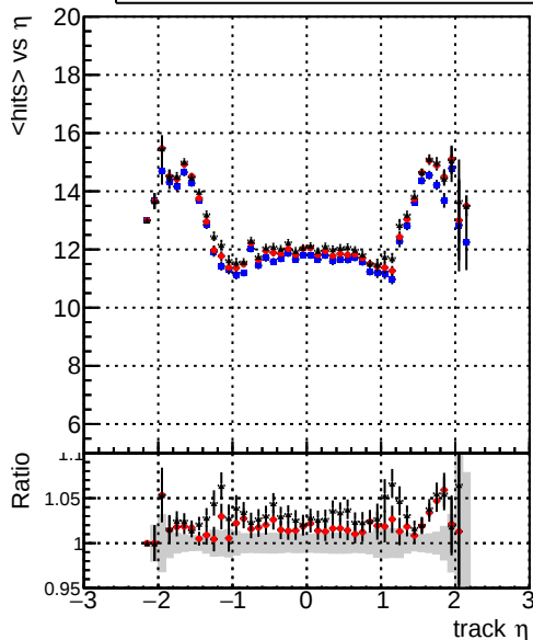
mean hits vs \eta Legend: DQMstep3_TT_CKF (blue), DQMstep3_TT_default (red), DQMstep3_TT_defaultNEWT203 (black)
