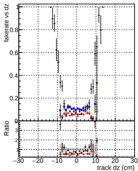
Fake rate vs d DOMstep3 TT CKF DOMstep3 default DOMstep3 defaultNEWT203
