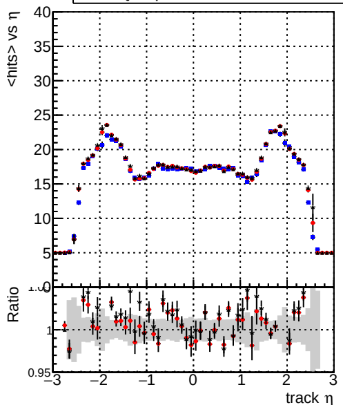
mean hits vs \eta — DQMstep3_TT_CKF — DQMstep3_TT_default — DQMstep3_TT_defaultNEWT203
