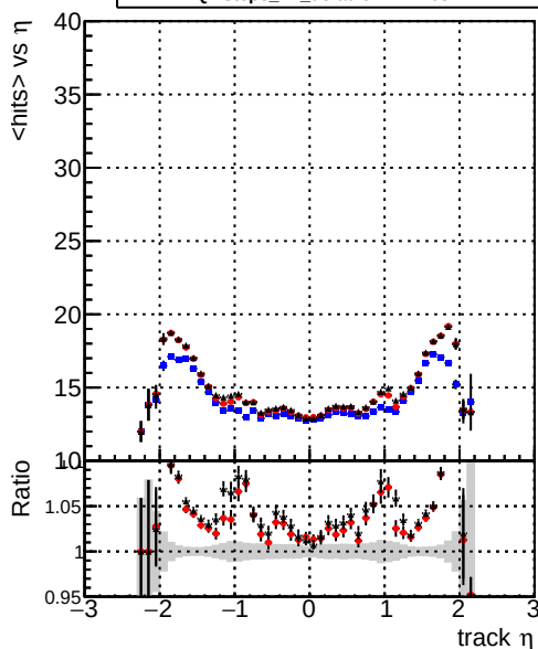
mean hits vs \eta — DQMstep3_TT_CKF — DQMstep3_TT_default — DQMstep3_TT_defaultNEWT203
