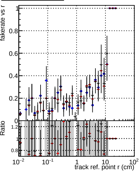
Fake rate vs v DOMstep3 TT CKF DOMstep3 TT default DOMstep3 TT defaultNEW203
