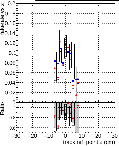
Fake rate vs verpos DOMstep3_TT_CKF DOMstep3_TT_default DOMstep3_TT_defaultNEW203
