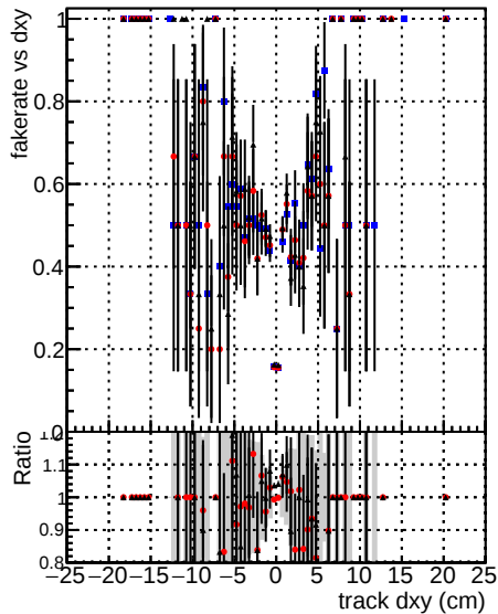
—●— DOMstep3 TT CKF —●— DOMstep3 default —●— DOMstep3 defaultNEW203
