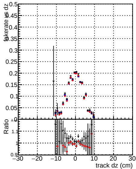
—●— DOMstep3 TT CKF —●— DOMstep3 default —●— DOMstep3 defaultNEW203
