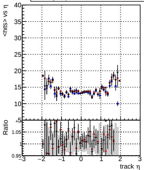
DQMstep3_TT_CKF DQMstep3_TT_default DQMstep3_TT_defaultNEWT203 mean hit
