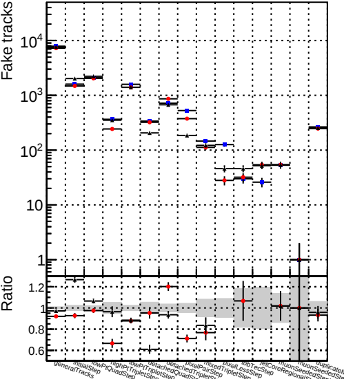
Number DQMstep3_TT_CKF DQMstep3_TT_default DQMstep3_TT_defaultNEWT203
