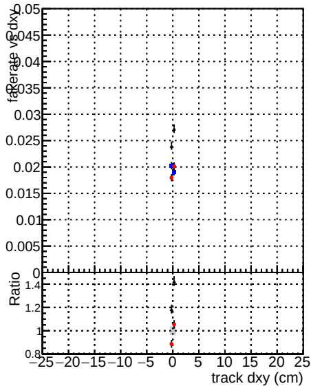
Fake rate vs d DOMstep3 TT CKF DOMstep3 TT default DOMstep3 TT defaultNEWT203
