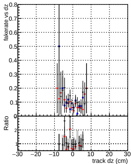
Fake rate vs dz DOMstep3 TT CKF DOMstep3 default DOMstep3 defaultNEW203
