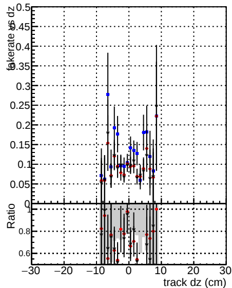
Fake rate vs dz DOMstep3 TT CKF DOMstep3 default DOMstep3 default NEWT203
