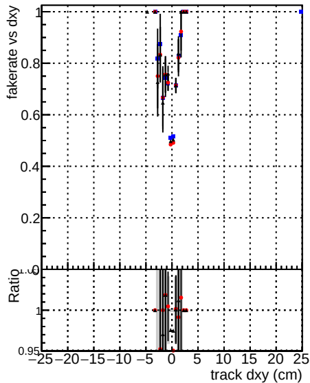
Fake rate vs d —●— DOMstep3 TT CKF —●— DOMstep3 TT default —●— DOMstep3 TT defaultNEW203
