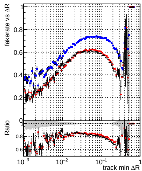
—●— DQMstep3 TT CKF —●— DQMstep3 TT default —●— DQMstep3 TT defaultNEW203
