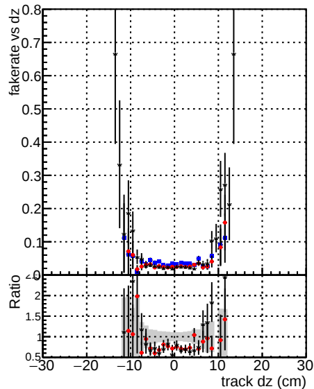
Fake rate vs dz DOMstep3 TT CKF DOMstep3 default DOMstep3 default
