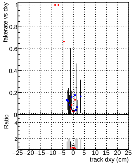
— DOMstep3 TT CKF — DOMstep3 TT default — DOMstep3 TT defaultNEWT203
