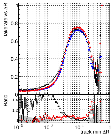
—●— DQMstep3_TT_CKF —●— DQMstep3_TT_default —●— DQMstep3_TT_defaultNEWT20
