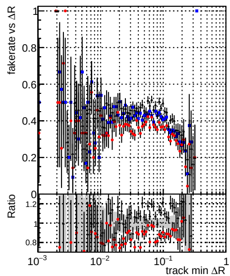
Legend: DQMstep3 TT CKF (blue squares) DQMstep3 TT default (red stars) DQMstep3 TT defaultNEW20 (black crosses)
