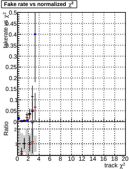
Fake rate vs. \chi^2 DOMstep3 TT CKF default DOMstep3 default NEWT20
