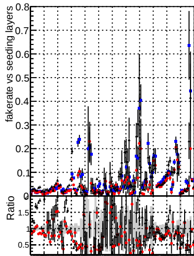
Fake rate vs. —●— DOMstep3 TT CKF —●— DOMstep3 default NEWT20
