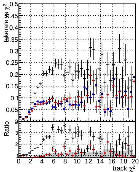
Fake rate vs. —●— DOMstep3 TT CKF —●— DOMstep3 default NEWT20
