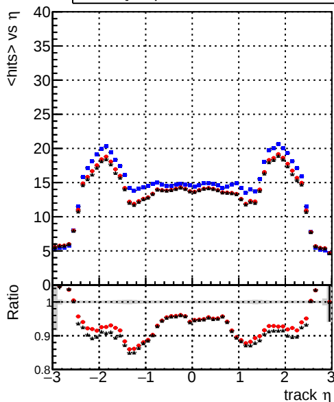
mean hits — DQMstep3_TT_CKF — DQMstep3_TT_default — DQMstep3_TT_defaultNEW20
