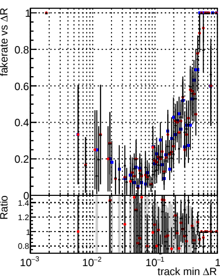
Fake rate vs \Delta R (track, jet) DQMstep3 TT CKF DQMstep3 TT default DQMstep3 TT defaultNEW20
