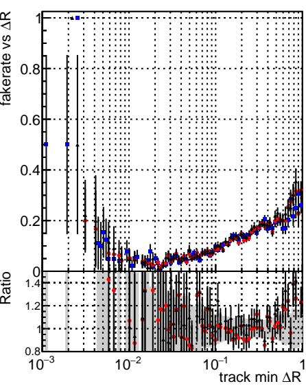
Fake rate vs —●— DQMstep3_TT_CKF —●— DQMstep3_TT_default —●— DQMstep3_TT_defaultNEW20
