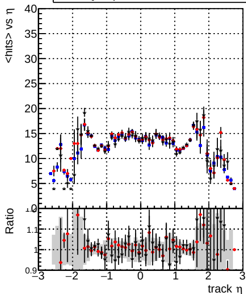
mean hit — DQMstep3_TT_CKF — DQMstep3_TT_default — DQMstep3_TT_defaultNEW20
