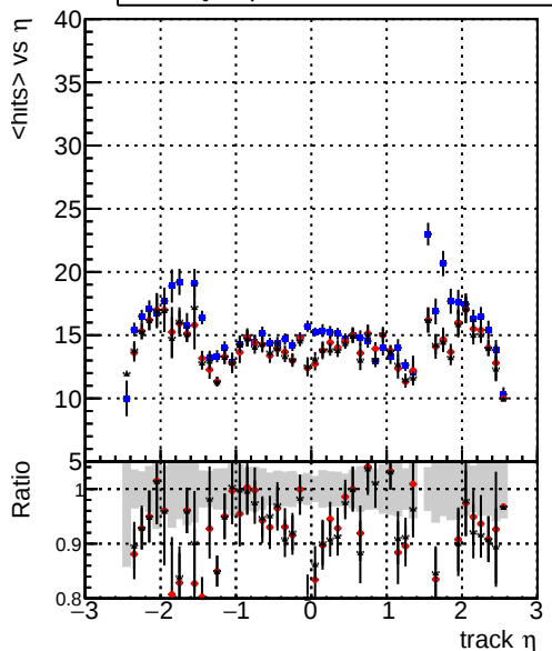
mean hit — DQMstep3_TT_CKF — DQMstep3_TT_default — DQMstep3_TT_defaultNEWT20
