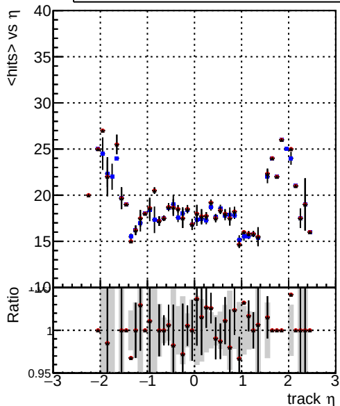
mean hit — DQMstep3_TT_CKF — DQMstep3_TT_default — DQMstep3_TT_defaultNEWT20
