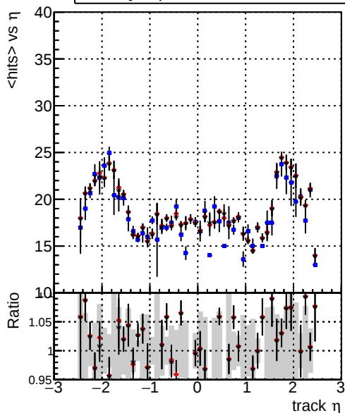
mean hits — DQMstep3_TT_CKF — DQMstep3_TT_default — DQMstep3_TT_defaultNEWT20
