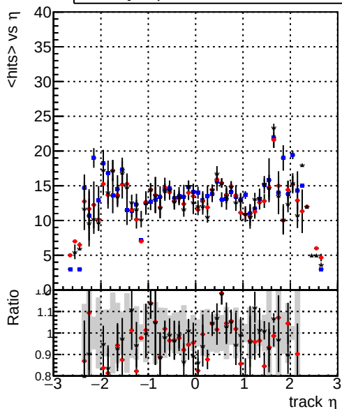
DQMstep3_TT_CKF DQMstep3_TT_default DQMstep3_TT_defaultNEWT20 mean hits
