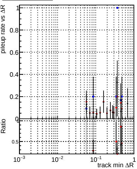
Legend: —●— DQMstep3_TT_CKF —●— DQMstep3_TT_default —●— DQMstep3_TT_defaultNEW20
