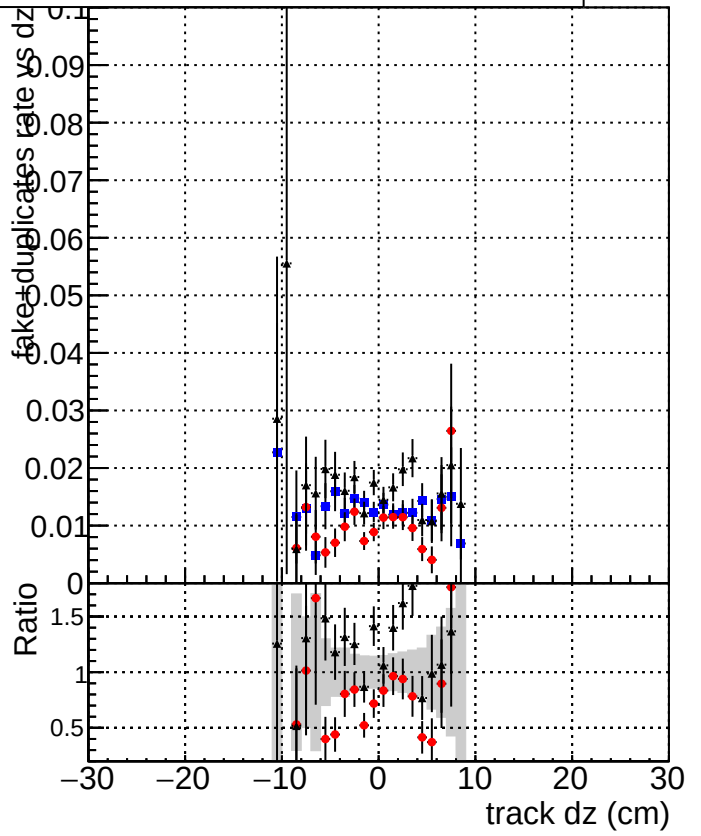
Legend for the bottom plot: DQMstep3_TT_CKF (blue squares) DQMstep3_TT_default (red circles) DQMstep3_TT_defaultNEWT20 (black triangles)
